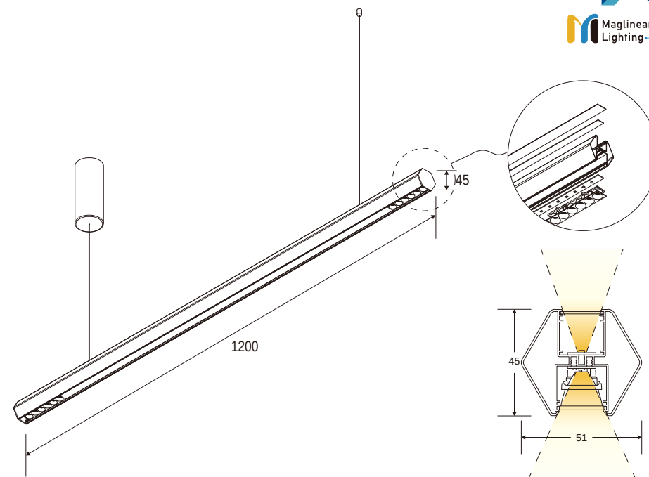
明装吊灯切面 Model: MAG-20-5145-APA
