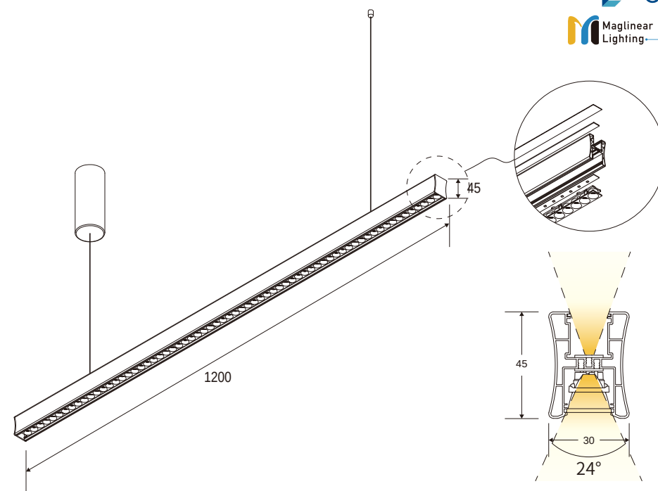
明装吊灯切面 Model: MAG-20-3045-A
