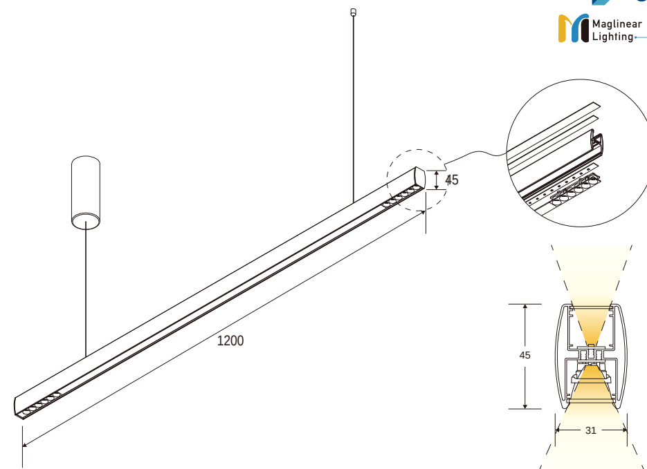
明装吊灯切面 Model: MAG-20-5145-APA
